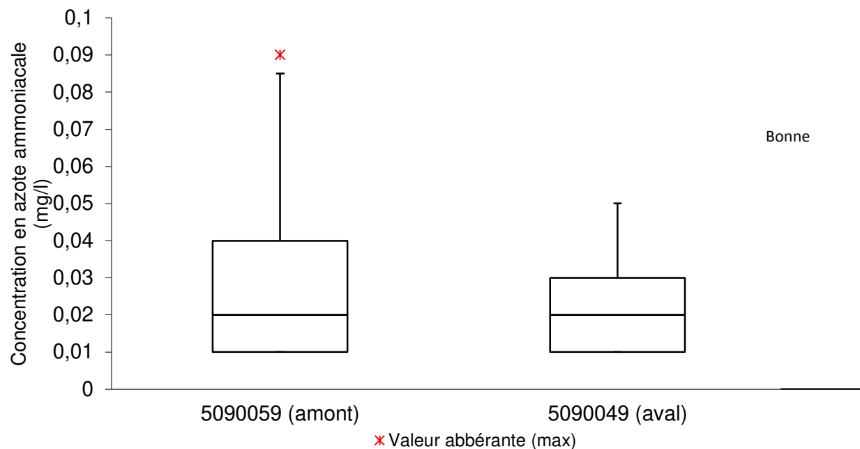
Figure 10 : Concentrations médianes en azote ammoniacal aux stations 05090059 et 05090049 en 2012.
