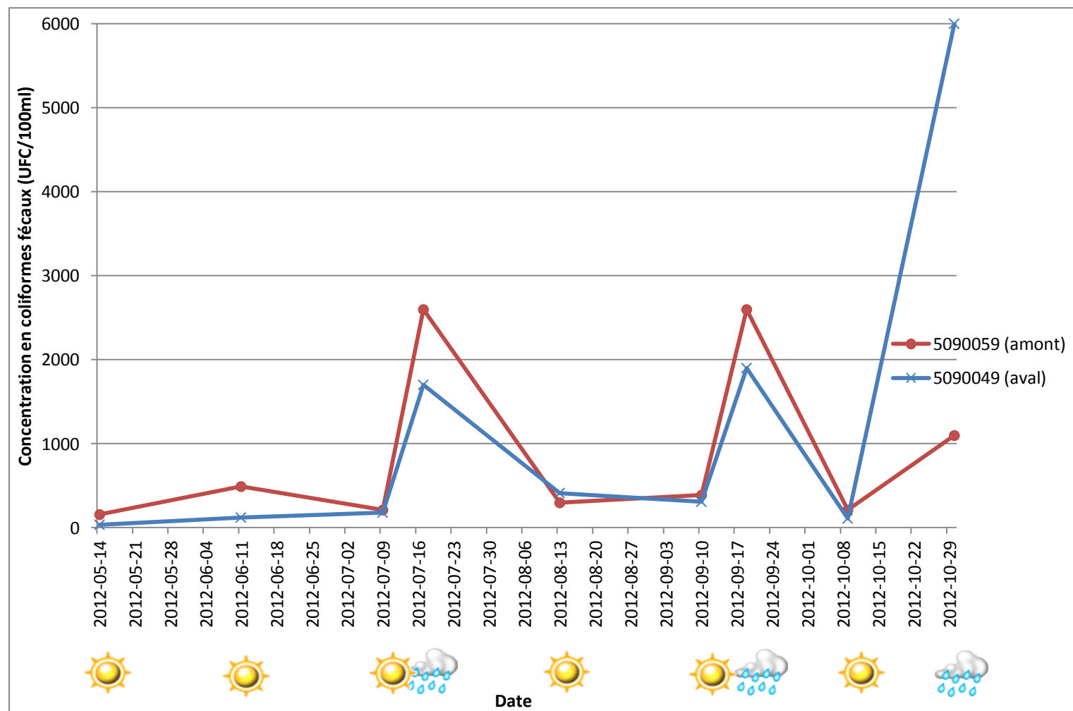
Figure 13 : Concentrations en coliformes fécaux mesurées aux stations 05090059 et 05090049 en 2012.
