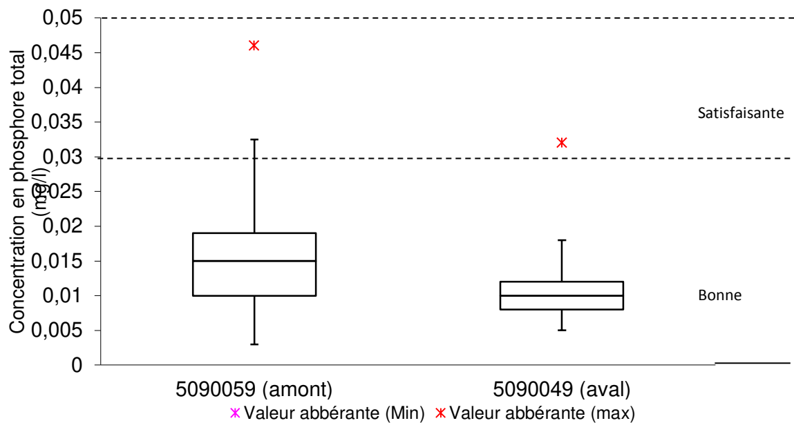
Figure 8 : Concentrations médianes en phosphore total aux stations 05090059 et 05090049 en 2012.
