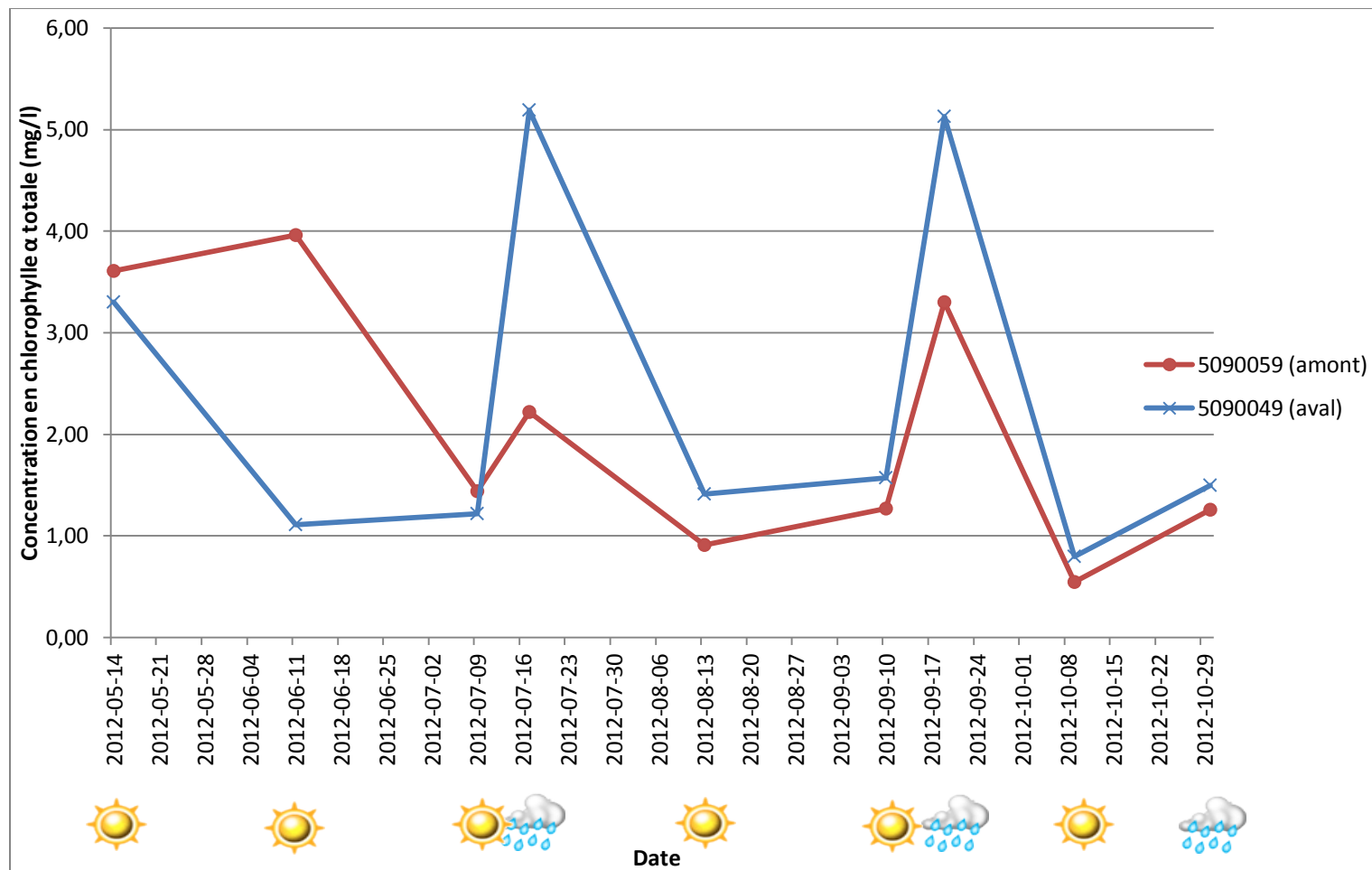
Figure 19 : Concentrations en chlorophylle \alpha totale mesurées aux stations 05090059 et 05090049 en 2012.
