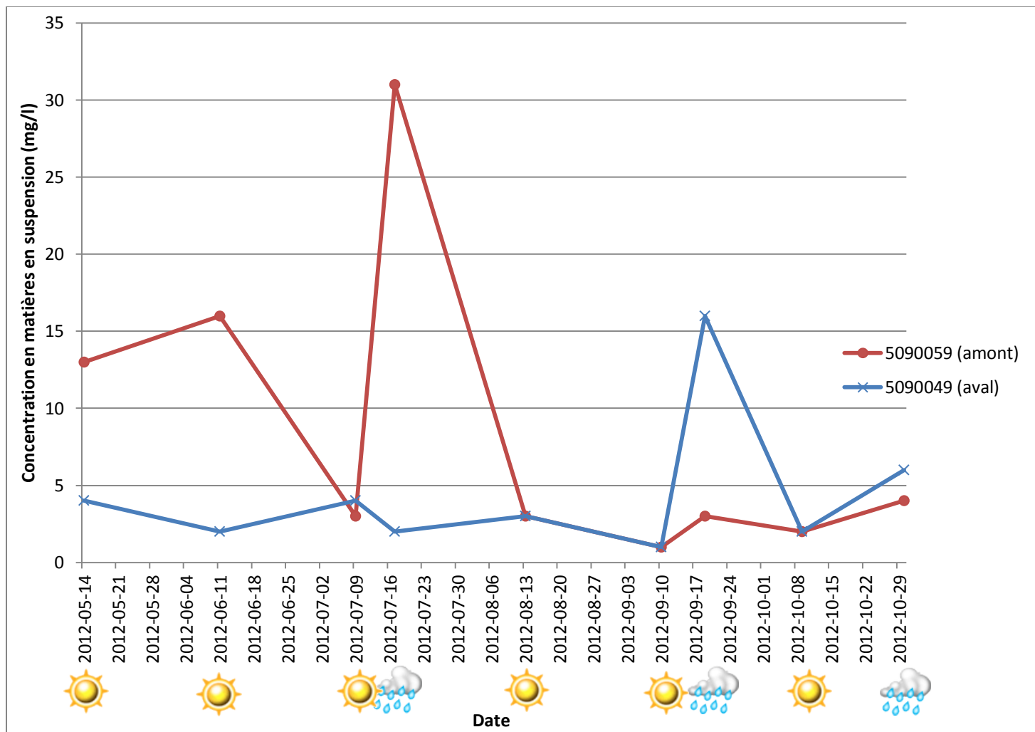
Figure 14 : Concentrations en matières en suspension mesurées aux stations 05090059 et 05090049 en 2012.
