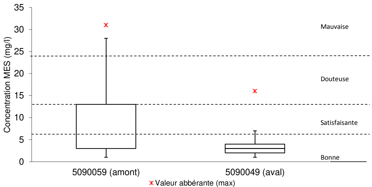
Figure 7 : Concentrations médianes en matières en suspension aux stations 05090059 et 05090049 en 2012.
