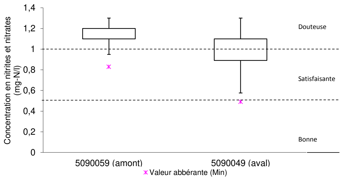
Figure 9 : Concentrations médianes en nitrites et nitrates aux stations 05090059 et 05090049 en 2012.
