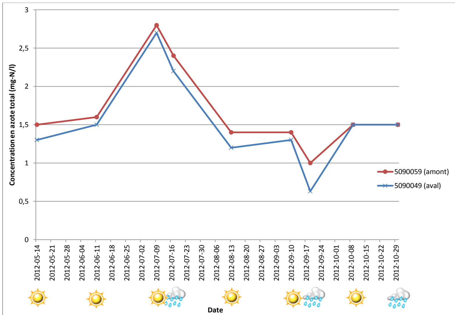
Figure 16 : Concentrations en azote total mesurées aux stations 05090059 et 05090049 en 2012.
