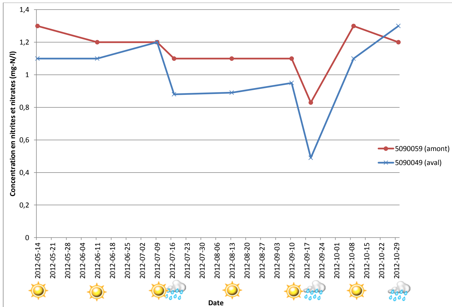
Figure 17 : Concentrations en nitrites et nitrates mesurées aux stations 05090059 et 05090049 en 2012.
