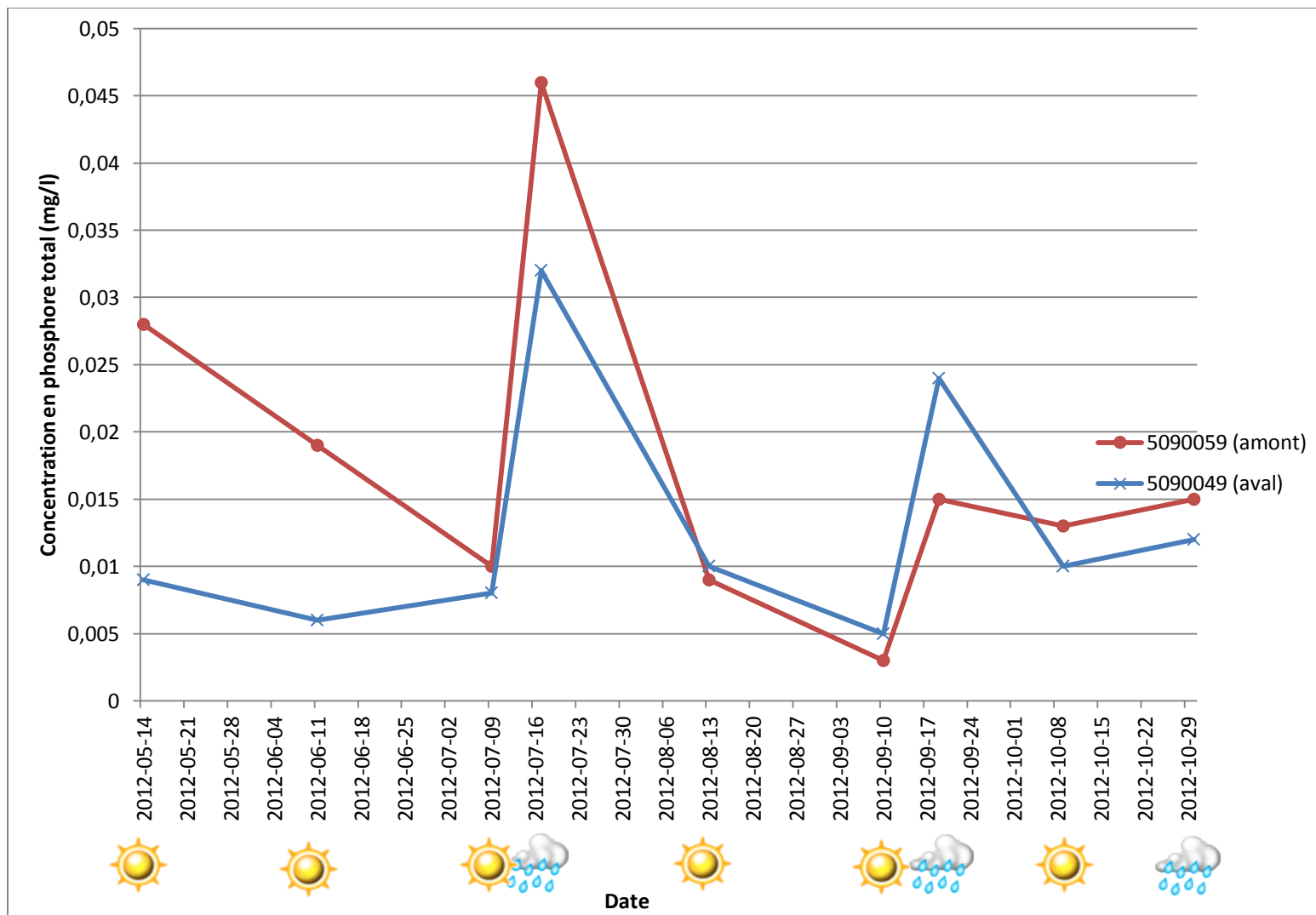
Figure 15 : Concentrations en phosphore total mesurées aux stations 05090059 et 05090049 en 2012.
