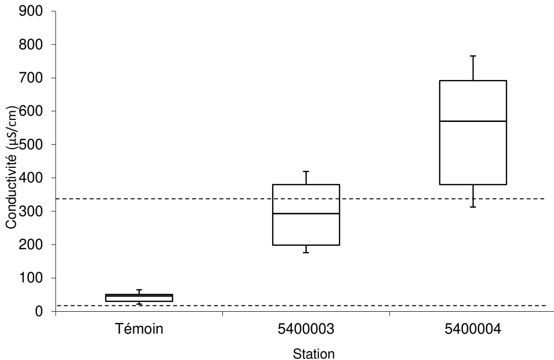
Figure 6: Données de conductivité collectées sur la rivière Beauport en 2011, de l'amont vers l'aval.
