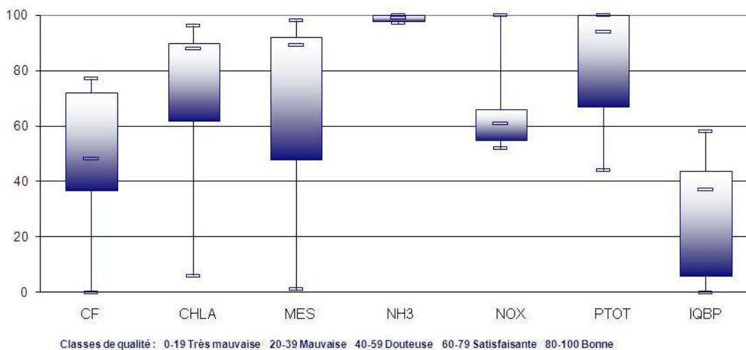
Figure 3 : Valeur de l'IQBP à la station 05400004 pour les périodes comprises entre le 9 mai et le 18 octobre 2011.
