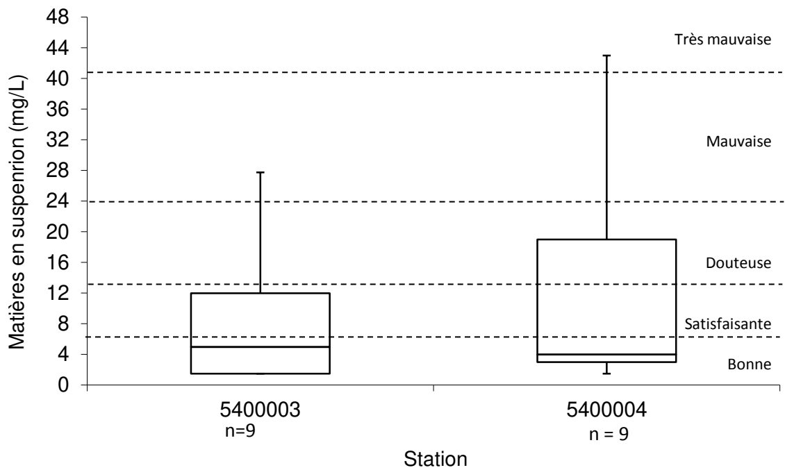
Figure 8 : Concentration en matières en suspension aux stations 05400003 et 05400004 en 2011.
