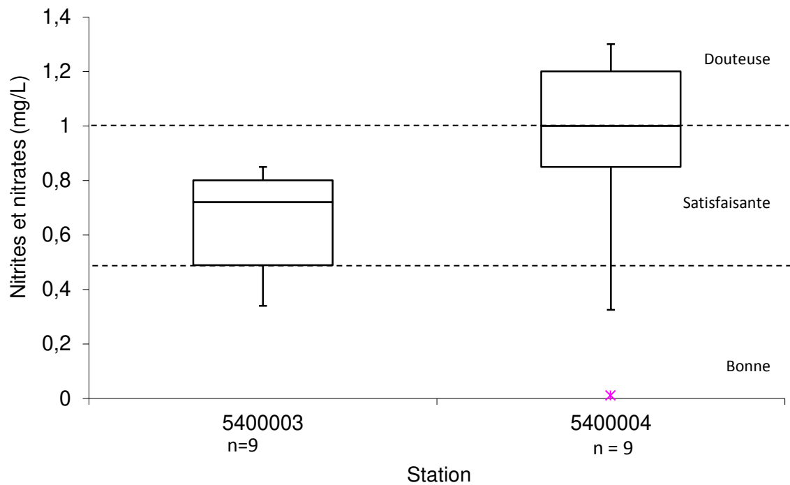
Figure 10 : Concentration en nitrites et nitrates aux stations 05400003 et 05400004 en 2011.
