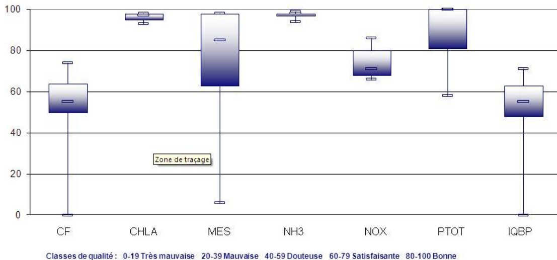
Figure 2 : Valeur de l'IQBP à la station 05400003 pour les périodes comprises entre le 9 mai et le 18 octobre 2011.
