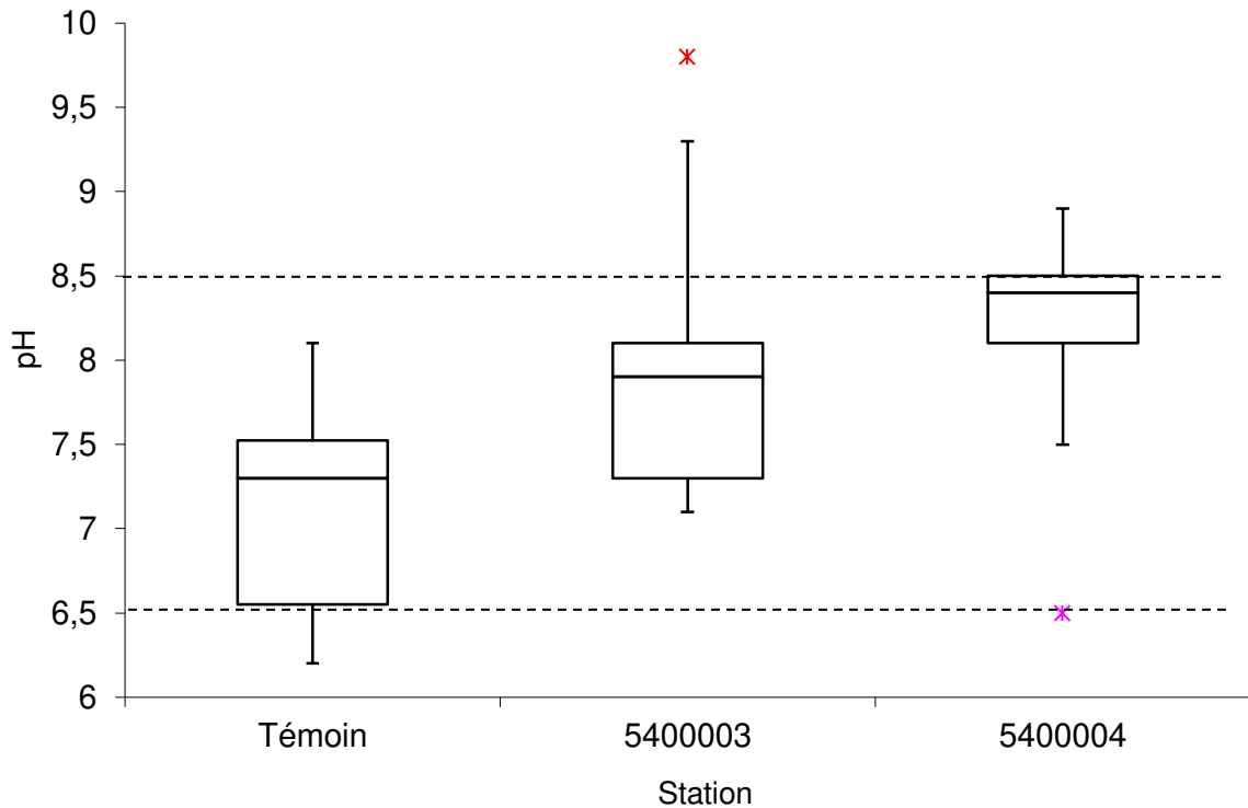
Figure 4 : Données de pH collectées sur la rivière Beauport en 2011, de l'amont vers l'aval.
