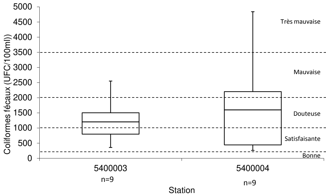
Figure 7 : Concentration en coliformes fécaux aux stations 05400003 et 05400004 en 2011.
