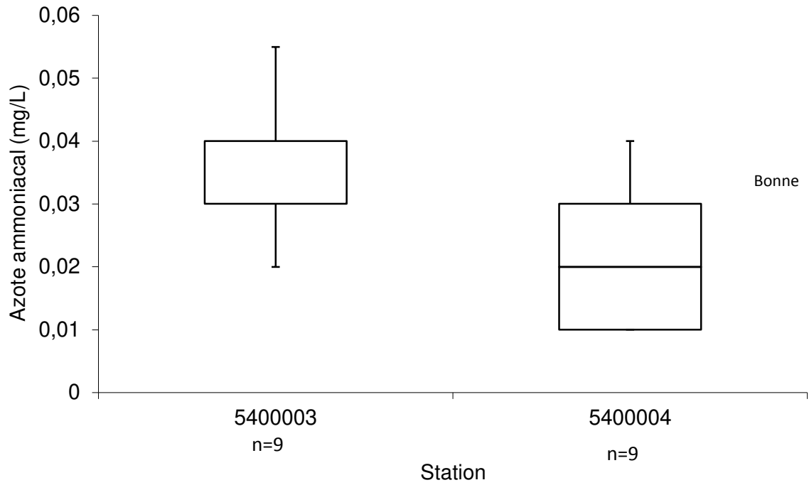
Figure 11 : Concentration en azote ammoniacal aux stations 05400003 et 05400004 en 2011.
