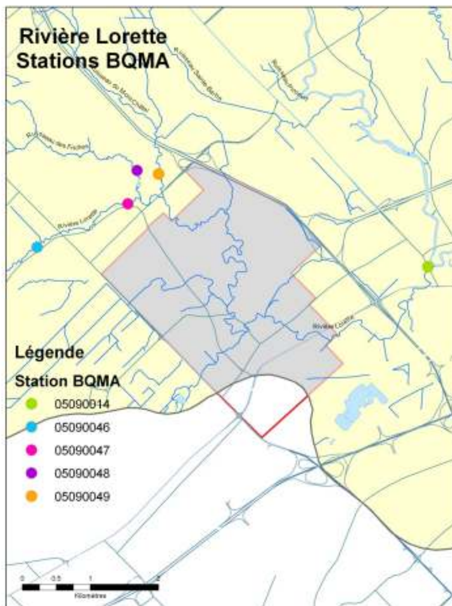
Figure 4 : Localisation des stations de la BQMA dans le bassin versant de la rivière Lorette
