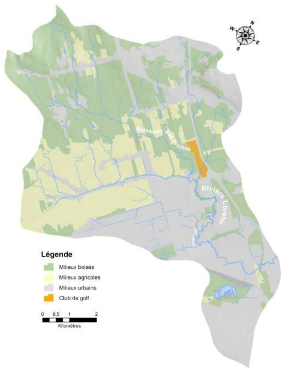
Figure 2 : Utilisation du sol du bassin versant de la rivière Lorette
