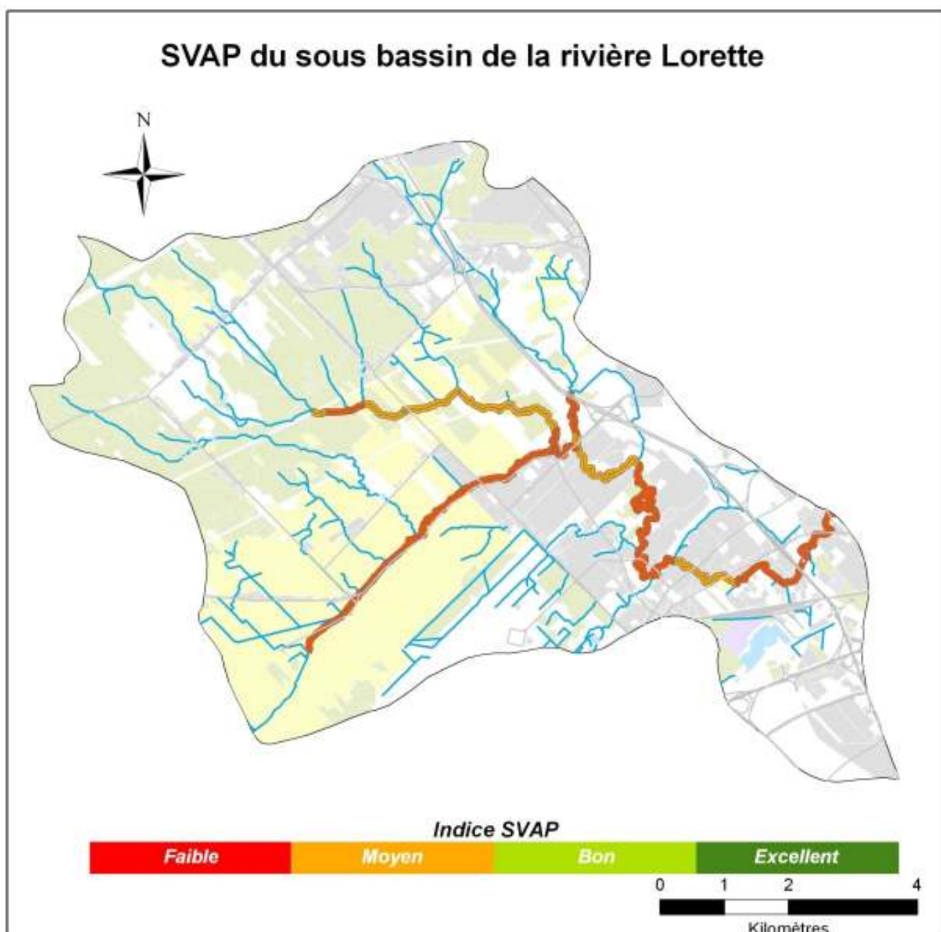
Figure 3 : Indice SVAP de la rivière Lorette
